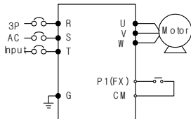
接线
