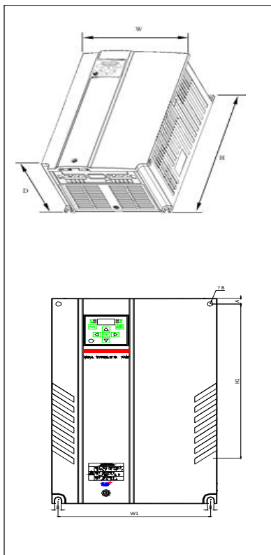
SV185iGxA-4 / SV220iGxA-4
