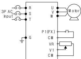
接线
